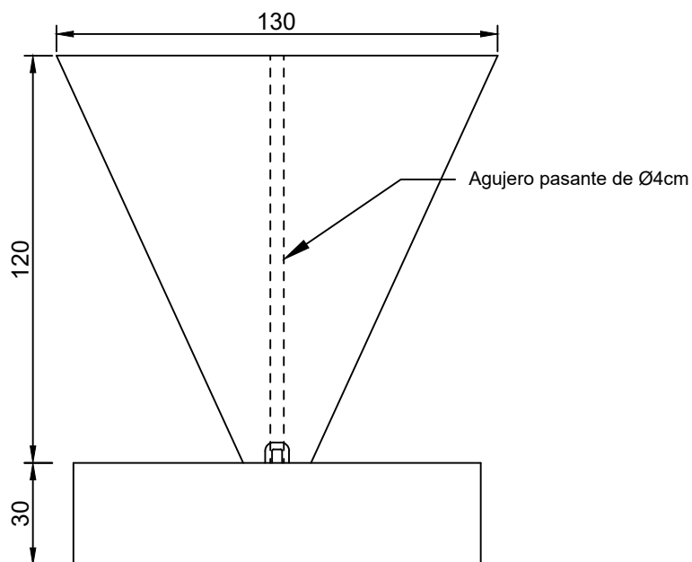
Alzado (cm) (1:2)
