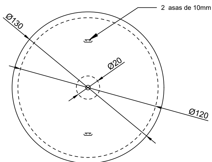
Planta (cm) (1:2)
