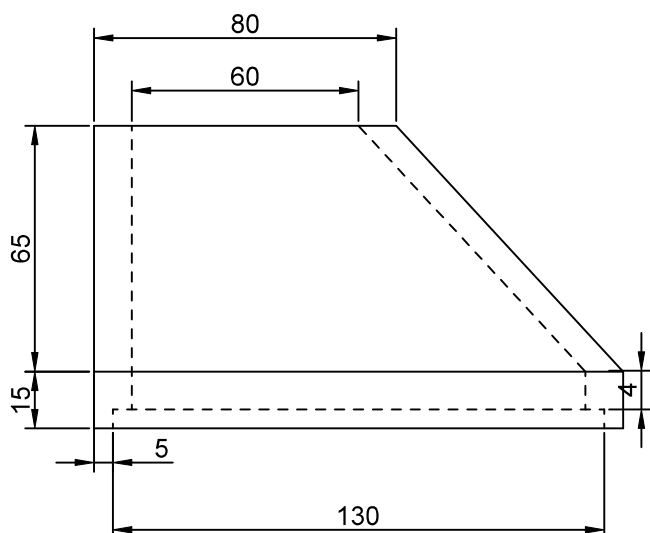
Alzado (cm) (1:2)
