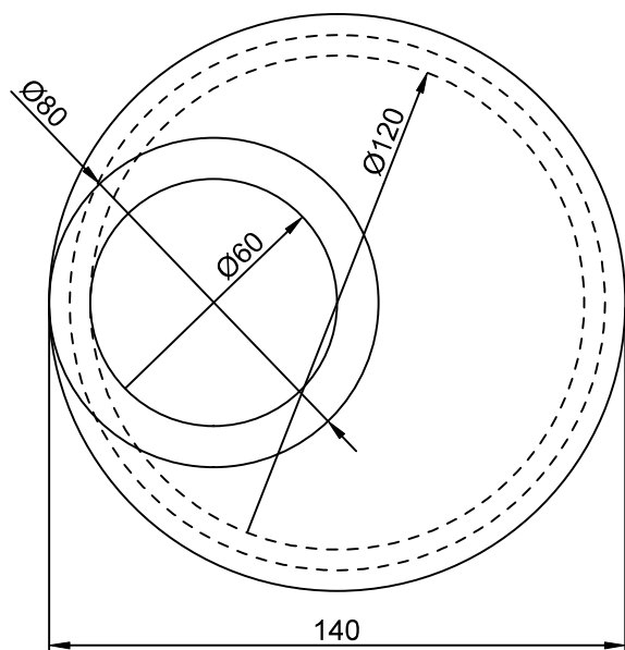
Alzado (cm) (1:2)
