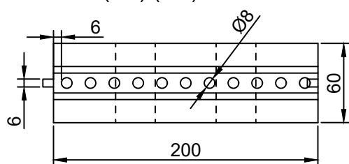
Planta (cm) (1:4)
