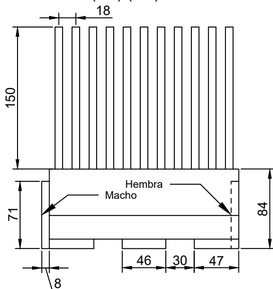
Alzado (cm) (1:4)
