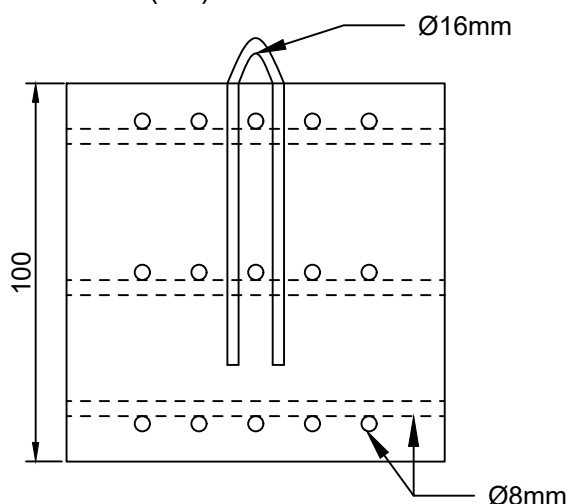
Perfil (cm) 1:2
