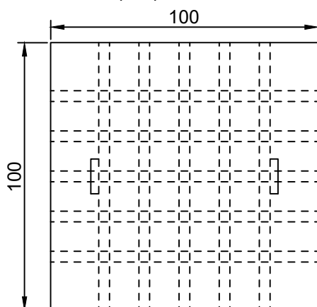
Planta (cm) 1:2
