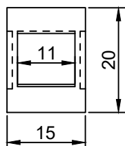
Planta (cm)
