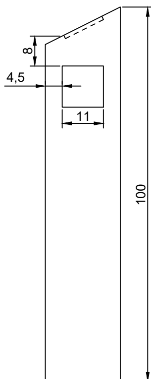
Perfil (cm)
