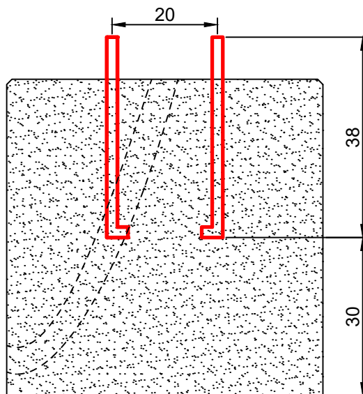
Corte A-A (cm)
