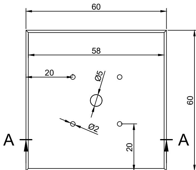
Planta (cm)
