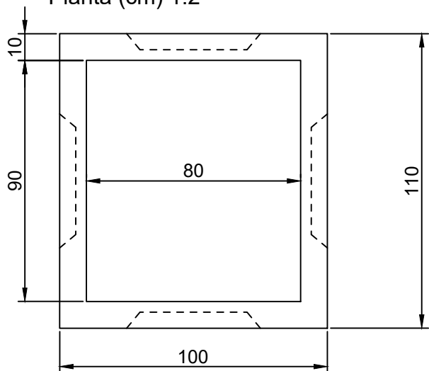
Planta (cm) 1:2
