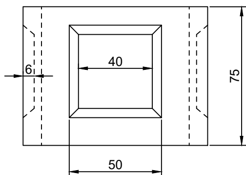
Perfil (cm) 1:2
