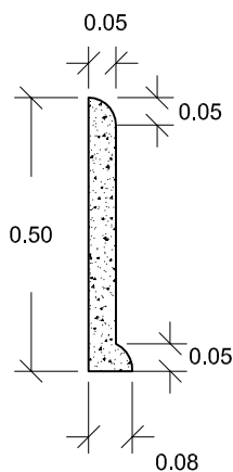
SECCION
