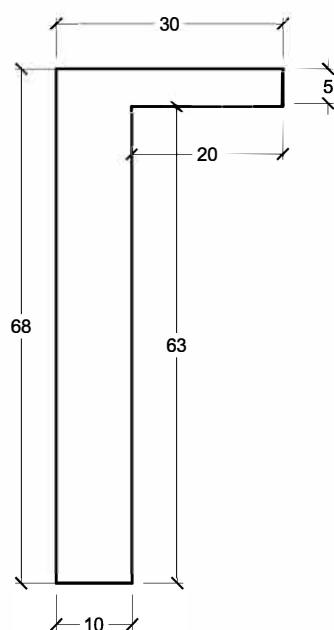
PERFIL
