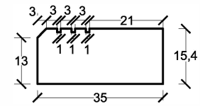
SECCIÓN a-a'
