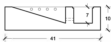
SECCION
