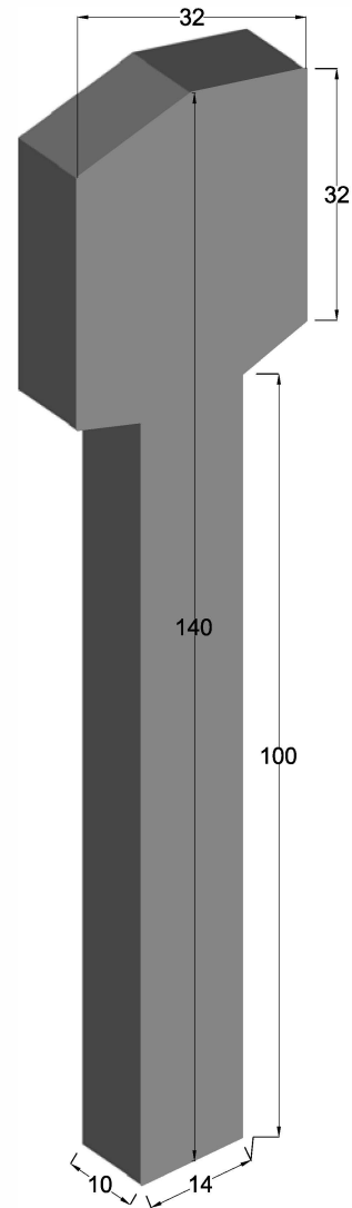
PERSPECTIVA cotas en cm.
