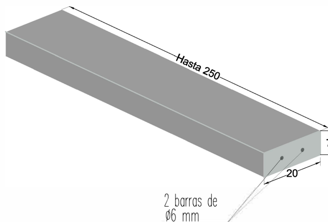
PERSPECTIVA cotas en cm.
