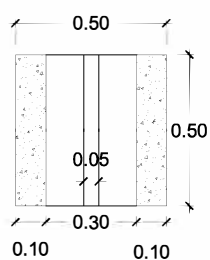
SECCIÓN a-a'
