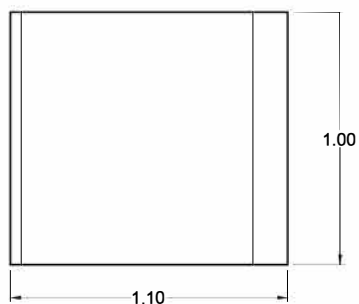
CANAL EN V 110 x 100
