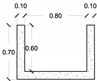
SECCION A-A'
