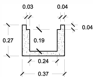
SECCIÓN a-a'
