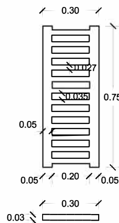
REJA DE HORMIGÓN armado de \phi 4 mm.
