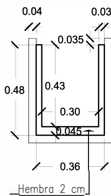
VISTA HEMBRA
