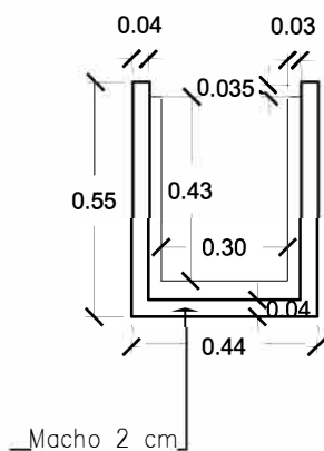
VISTA MACHO
