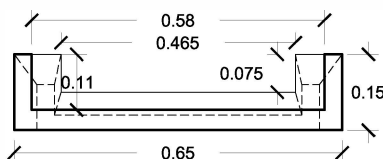
VISTA B
