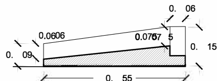
SECCION A-A'
