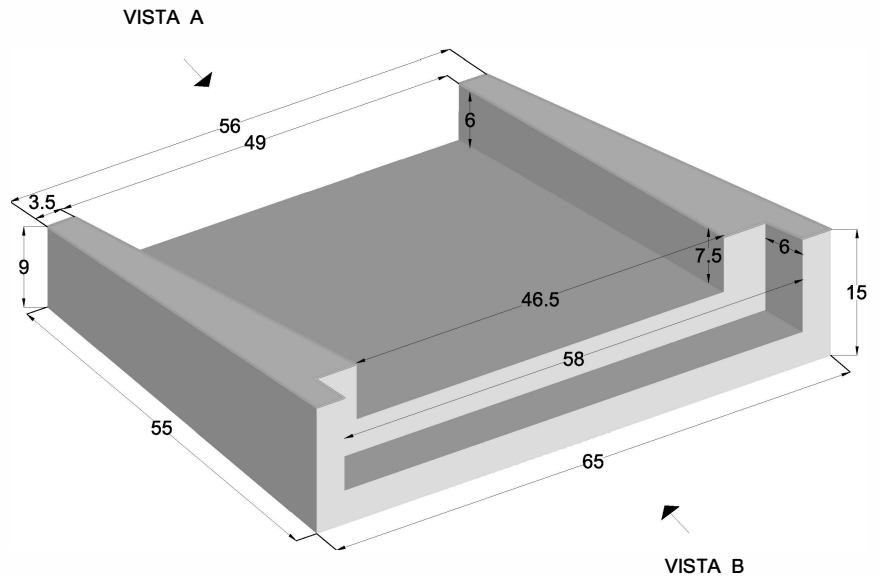
PERSPECTIVA cotas en cm.
