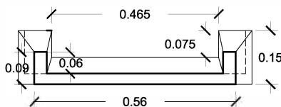
VISTA A
