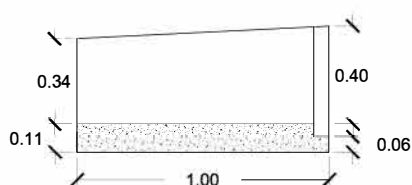
SECCION A-A'
