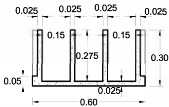
SECCION a-a'
