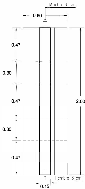
VISTA PLANTA
