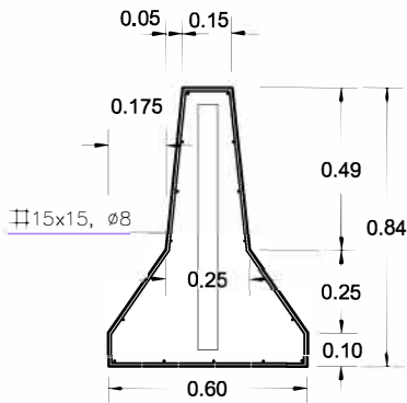
VISTA PERFIL
