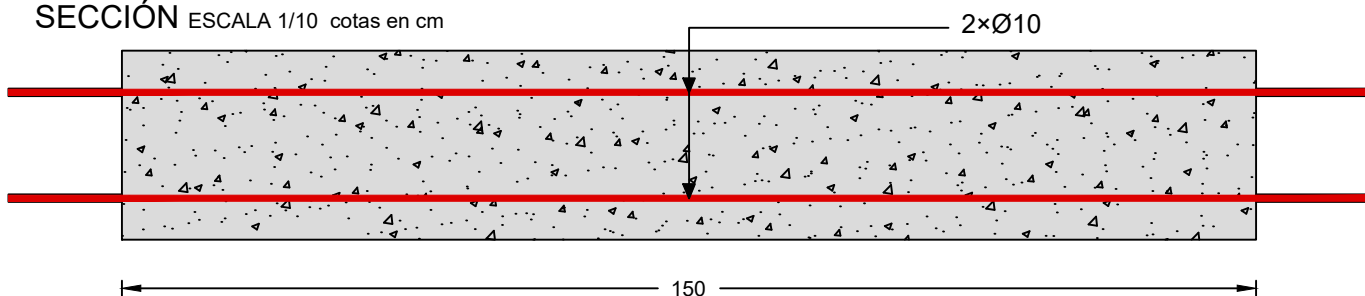
SECCIÓN ESCALA 1/10 cotas en cm
