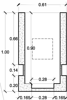
SECCION b-b'
