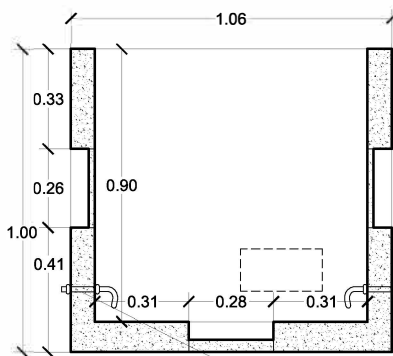
SECCION a-a'
