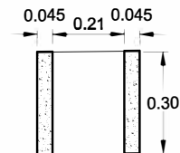
SECCION b-b'
