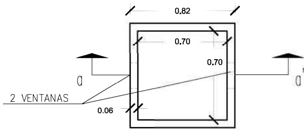
VISTA EN PLANTA
