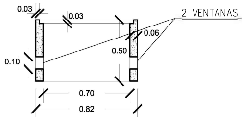
SECCION a-a'
