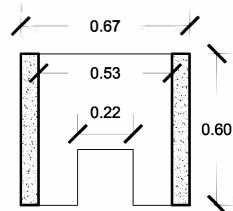
SECCION a-a'
