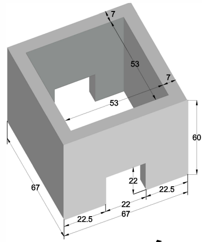
VISTA A
