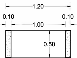
SECCION a-a'
