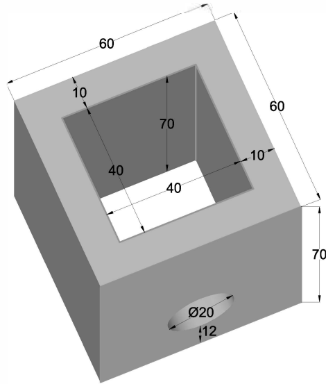
ARQUETA SIN FONDO cotas en cm.
