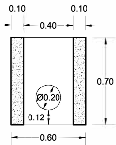
SECCION a-a' ARQ. SIN FONDO
