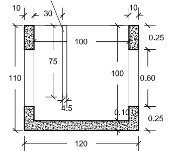
SECCION
