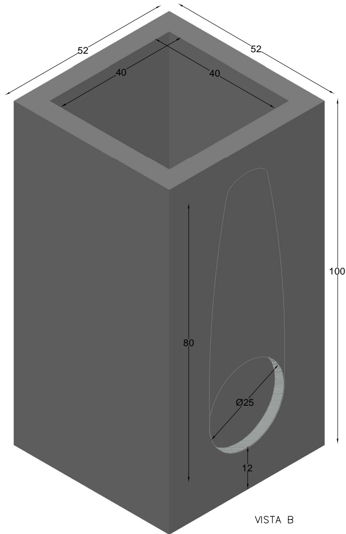
PERSPECTIVA cotas en cm.
