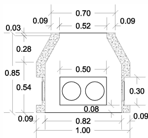
SECCION A-A'
