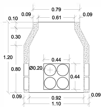
SECCION B-B'
