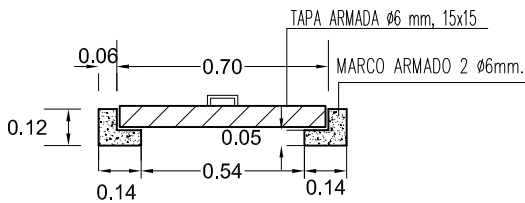
SECCION A-A'
