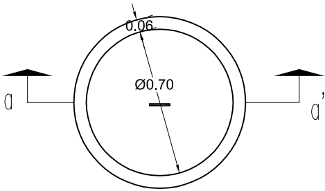
PLANTA DE MARCO Y TAPA
