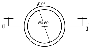
PLANTA DE MARCO Y TAPA
