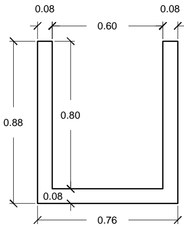
VISTA A
