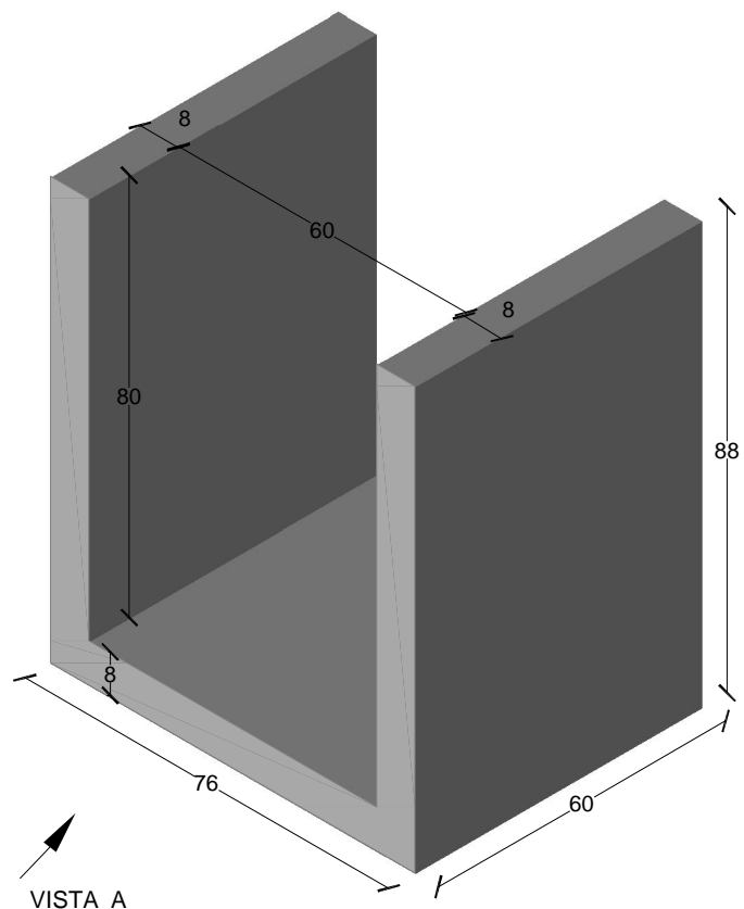
VISTA A
