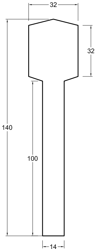
ALZADO
