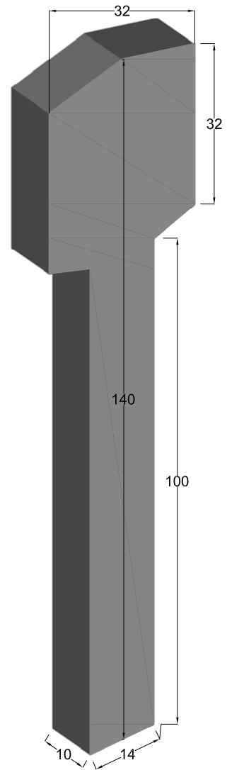
PERSPECTIVA cotas en cm.
