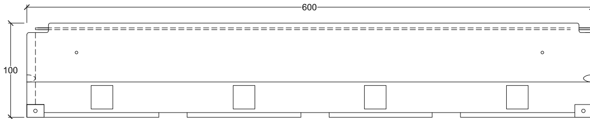
VISTA ALZADO
