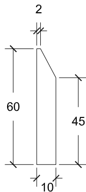
PERFIL
