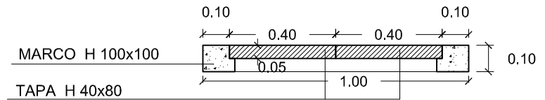
SECCION
