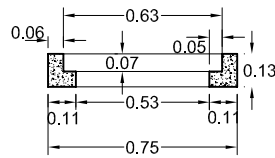
MARCO DE HORMIGÓN SECCION a-a' MARCO ARMADO 2 \phi 6 mm.
