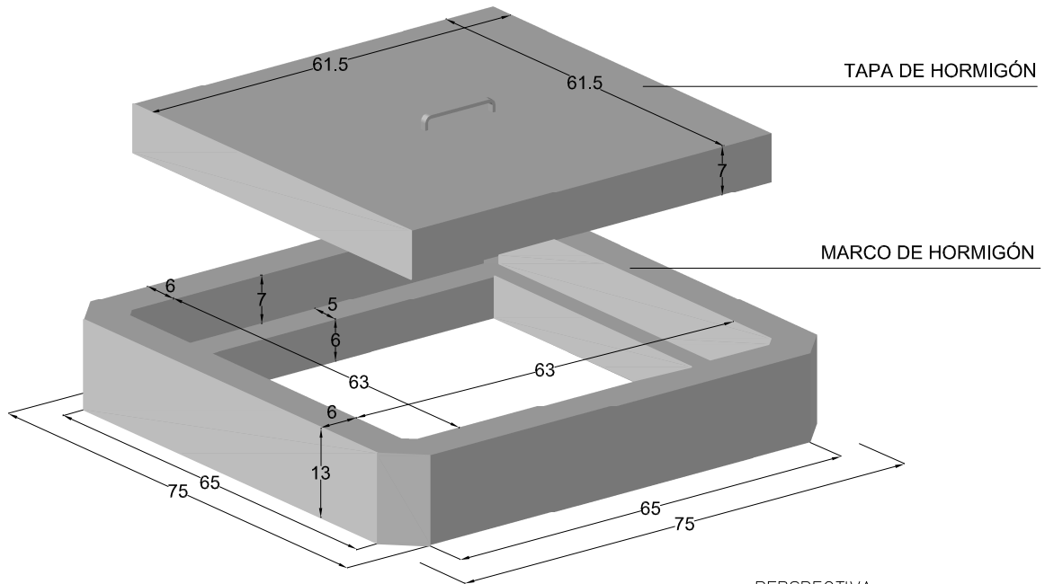
PERSPECTIVA cotas en cm.
