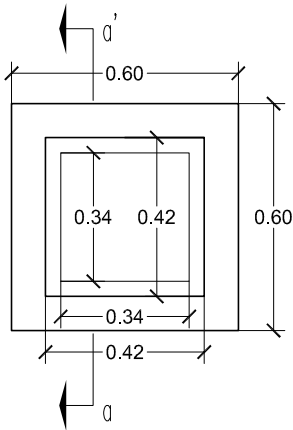
MARCO DE HORMIGÓN PLANTA
