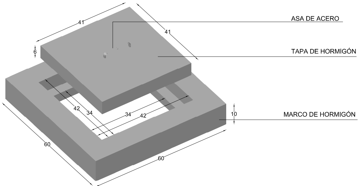
PERSPECTIVA cotas en cm.
