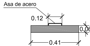
TAPA DE HORMIGÓN
