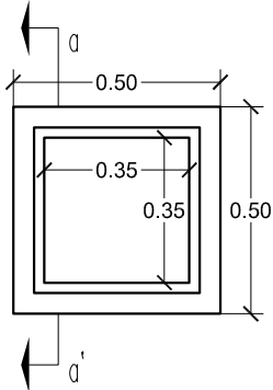
MARCO DE HORMIGÓN PLANTA
