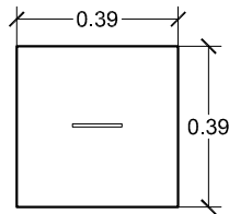
TAPA DE HORMIGÓN TAPA ARMADA \varnothing 6 mm, 15x15
