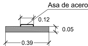
TAPA DE HORMIGÓN TAPA ARMADA \varnothing 6 mm, 15x15
