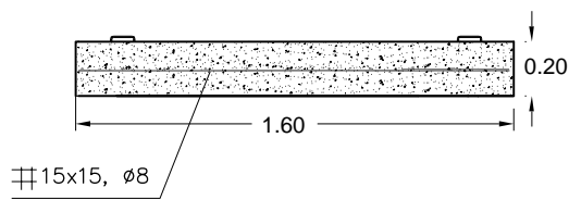
SECCION a-a'
