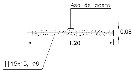
SECCION a-a'
