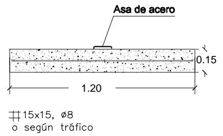
SECCION a-a'
