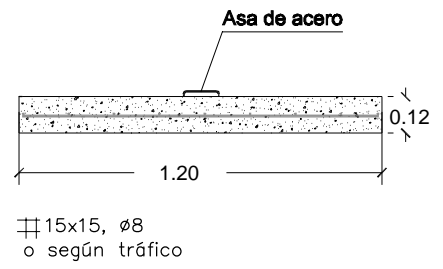
SECCION a-a'
