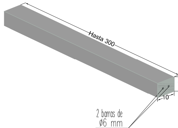
PERSPECTIVA cotas en cm.
