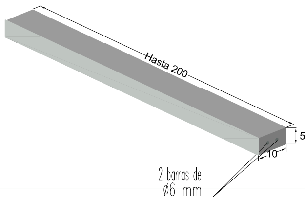
PERSPECTIVA cotas en cm.
