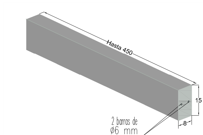
PERSPECTIVA cotas en cm.
